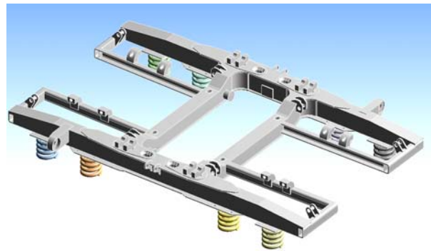
Рис. 8. Модель рами візка
