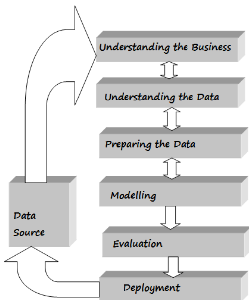
Fig. 5 CRISP DM-PROCESS
