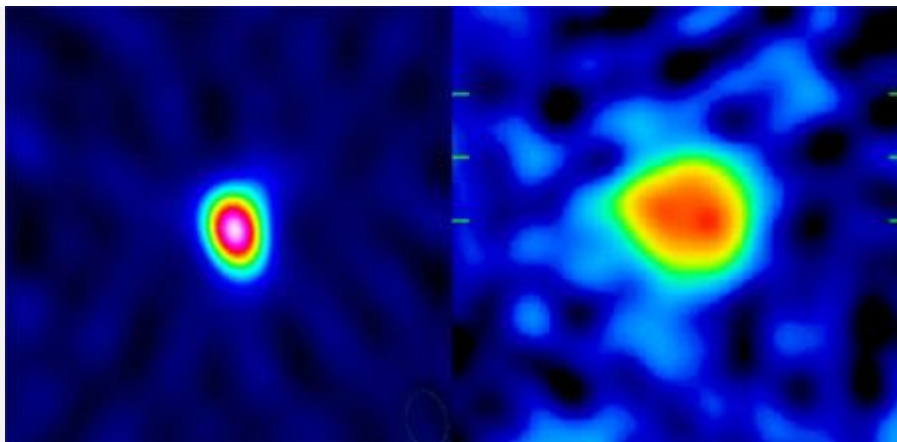
Sn1987/Betelgeuse
