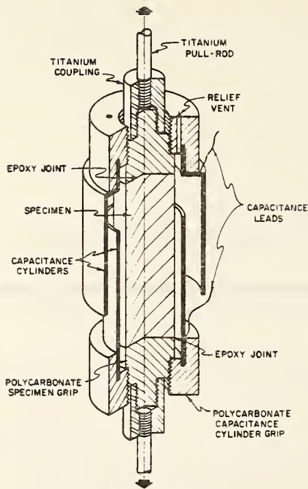
Tensile
