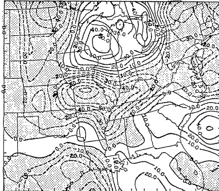
500 mb
