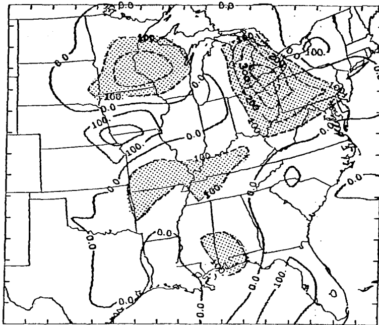
0600 GMT, 24 April
