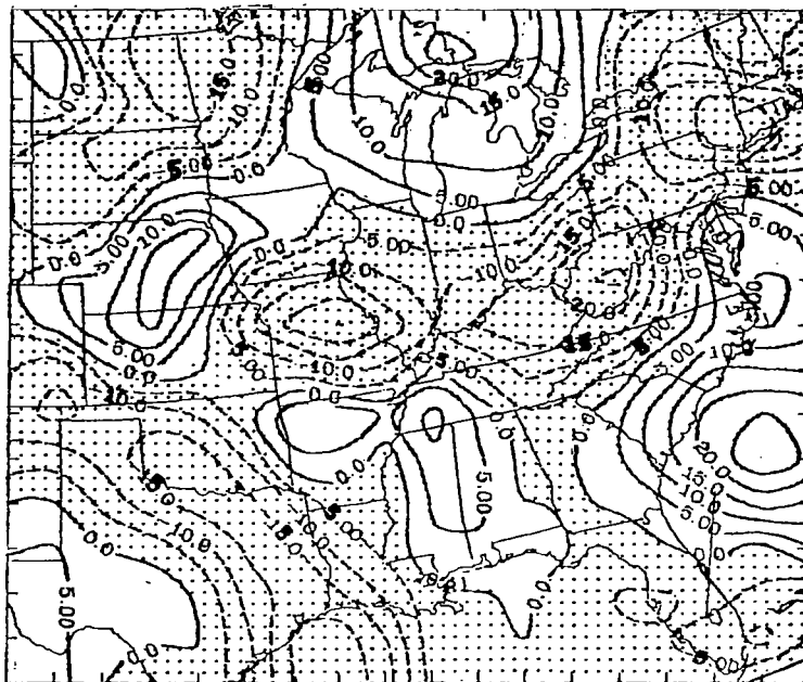
850 mb
