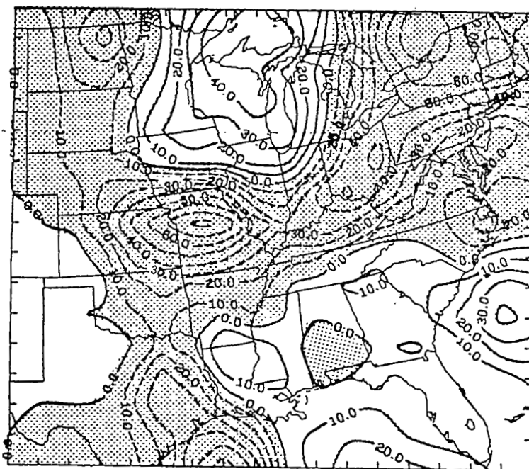
500 mb
