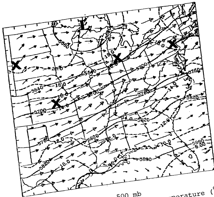
500 mb
