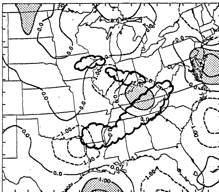
1200 GMT, 25 April b. 600 mb
