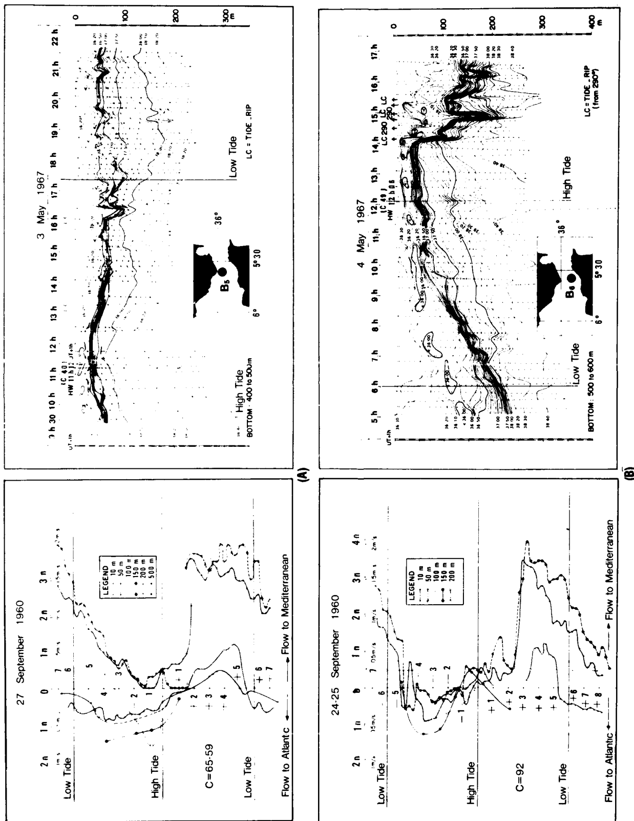
Figure 5 Tidal current speed and direction variations and salinity depth variations for a north and south point in the Strait of Gibraltar (from Calypso, 1960 and J. Charcot, 1967). The current graphs are arranged similar to Figure 3. The abscissa of the salinity graphs is a time presentation arranged in units of hours (after Lacombe, Richez, 1982; 1984). Vitesse du courant de marée longitudinal aux points B5 et B6 des 3 et 4 mai 1967 (J. Charcot). La présentation des courbes de courants est identique à celle de la figure 3. L'abscisse des courbes de salinité représente le temps en heures (d'après Lacombe, Richez, 1982; 1984).
