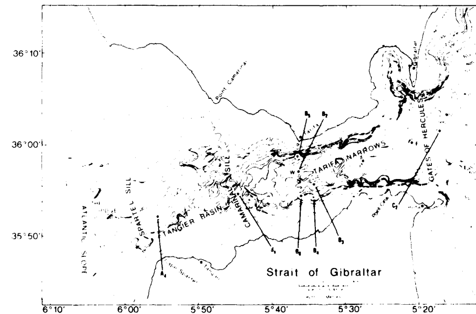
Figure 1 Bathymetry of the Strait of Gibraltar (modified by Armi and Farmer, 1985, from Lacombe and Richez, 1982 and from Giermann, 1961). Bathymétrie du détroit de Gibraltar (modifié par Armi et Farmer, 1985, d'après Lacombe et Richez 1982 et d'après Giermann, 1961).
