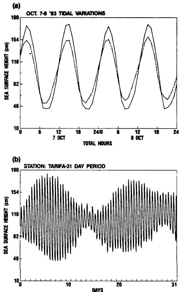
Figure 2 Hourly tide-height variations for (a) forty-eight hours for Tarifa (solid line) and Ceuta (dashed line) and for (b) a 31-day period for Tarifa (tide observations furnished by the Instituto Español de Oceanografía, Madrid, Spain). Courbes de marée (a) pour les 7 et 8 octobre 1983, à Tarifa (trait plein) et à Ceuta (tireté) et (b) pendant le mois d'octobre 1983 à Tarifa (documents fournis par l'Institut Espagnol d'Océanographie de Madrid).
