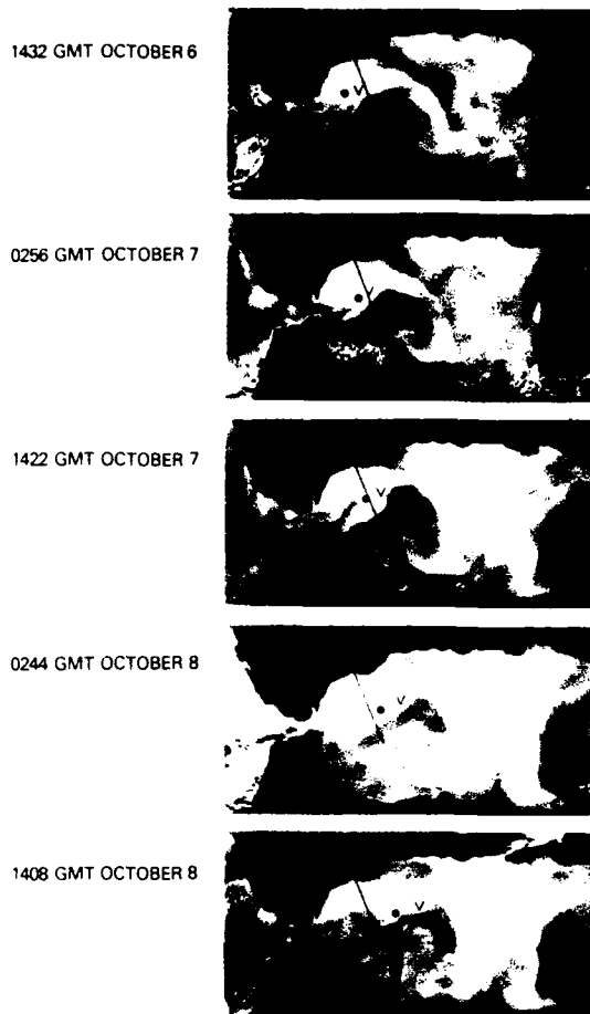
Figure 11 Cyclic emission of cold water features from the eastern end of the Strait of Gibraltar and their rotation about the Alboran gyre (La Violette, 1984). Émission cyclique de taches d'eau froide à partir de l'extrémité orientale du détroit et leur rotation autour de la Mer d'Alboran (La Violette, 1984).
