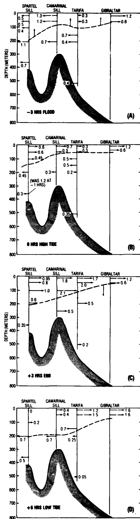
Figure 10 Tidal current speed and direction variations with depth along the axis of the Strait of Gibraltar for a constructed tide cycle. The dashed line represents the depth of the Atlantic water/Mediterranean water interface (from September 1960 ship data). Variations en fonction de la profondeur de la vitesse et de la direction des courants de marée le long de l'axe du détroit de Gibraltar, pour un cycle de marée reconstitué. La ligne en tirets représente la profondeur de l'interface entre eau atlantique et eau méditerranéenne (données de septembre 1960, Calypso).
