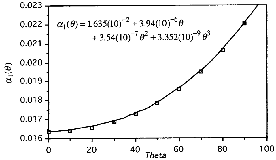
Figure 4.6.5 SVO Compensator Parameter \alpha_1(\theta)
