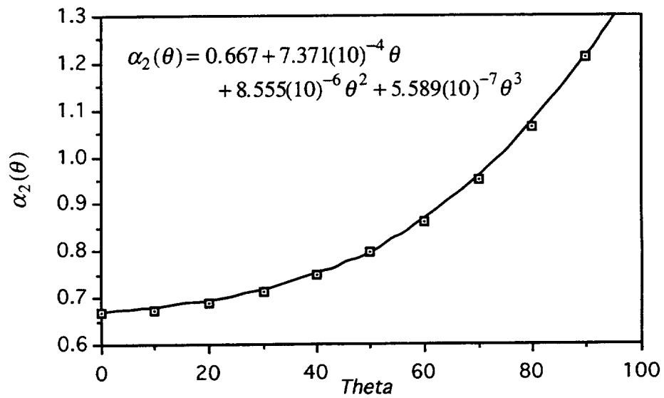
Figure 4.6.6 SVO Compensator Parameter \alpha_2(\theta)
