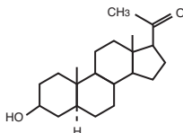
Iso-allopregnanolone
