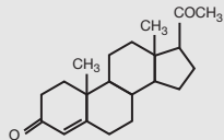
Progesterone
