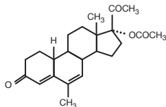
Nomegestrol acetate
