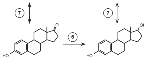
Estrone
