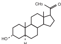
Allopregnanolone
