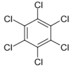
Hexachlorobenzene (HCB)
