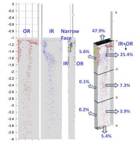
(d) Argon-steel flow, 400 \mu\text{m} slag particle
