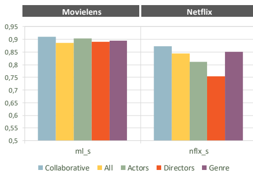
MAE - Movielens & Netflix
