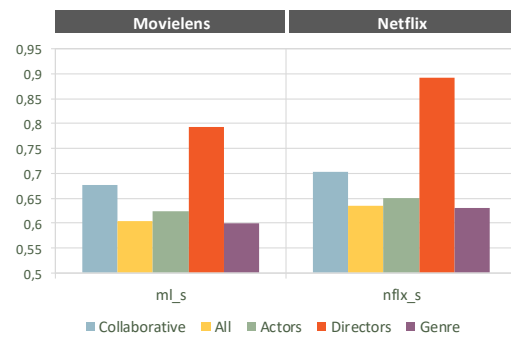
Precision - Movielens & Netflix
