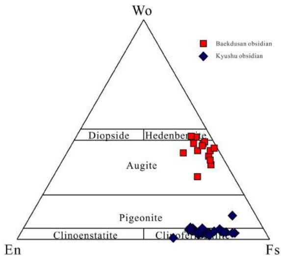
Figure 5. CaSiO_3(Wo) - MgSiO_3(En) - FeSiO_3(Fs) discrimination of clinopyroxene.
