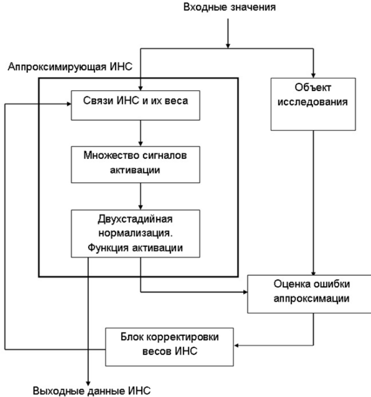
Рис. 1. Общая схема процесса обучения ИНС
