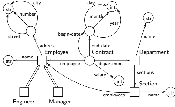
Fig. 2. A schema graph
