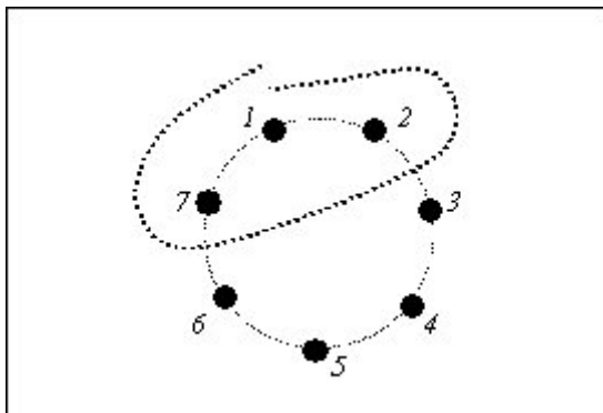
Fig. 2. Le cercle virtuel pour un essaim de sept particules. Le groupe d'information de taille trois de la particule 1 est composé des particules 1, 2 et 7.
