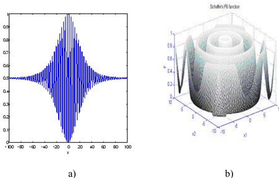
Fig. 1. Allure de la fonction de test F6. a) Représentation à une dimension dans le domaine [-100, 100]. b) Représentation à deux dimensions dans le domaine [-10, 10].
