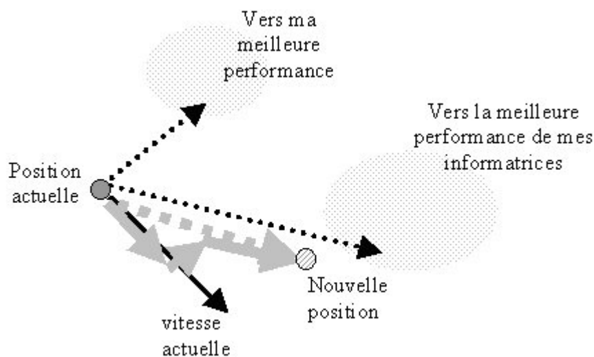
Fig. 3. Schéma de principe du déplacement d'une particule. Pour réaliser son prochain mouvement, chaque particule combine trois tendances : suivre sa vitesse propre, revenir vers sa meilleure performance, aller vers la meilleure performance de ses informatrices.
