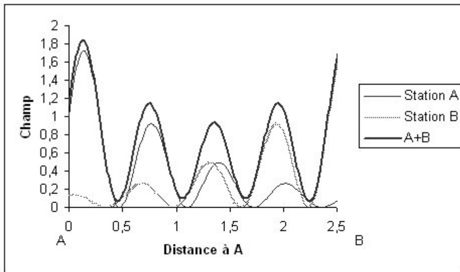
Fig. 4. Entre les deux stations A et B, à un instant donné, les valeurs des champs reçus se répartissent selon des sinusoides amorties. La distance entre les stations (ici 2,7 km) n'étant pas en rapport simple avec la longueur d'onde, le point où le champ total est minimum n'est pas facilement calculable.
