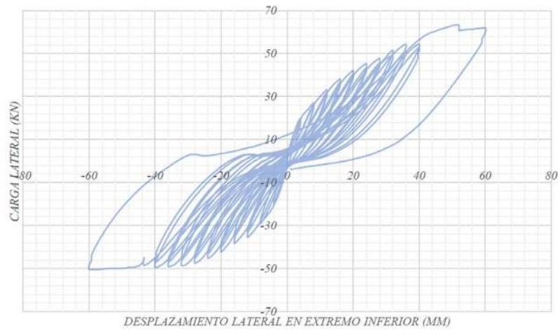
Figura 9. Respuesta de viga VE-02 sometida a cargas cíclicas Fuente: Elaboración propia
