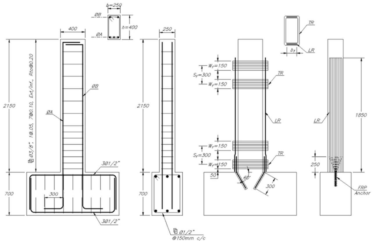
Figura 2. Detalles del refuerzo interno y externo de las vigas ensayadas Fuente: Elaboración propia
