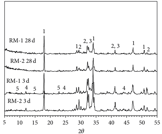
(1) \text{Ca}(\text{OH})_2 (2) \text{C}_3\text{S} (3) \text{C}_2\text{S} (4) \text{C}_4\text{AF} (5) \text{Ca}_6\text{Al}_2(\text{SO}_4)_3 \cdot 32\text{H}_2\text{O}
