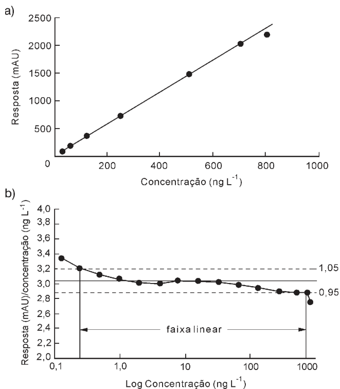
Figura 1. Determinação gráfica das curvas de linearidade através da: (a) curva analítica clássica; (b) gráfico da razão sinal/concentração vs. concentração em escala logarítmica
