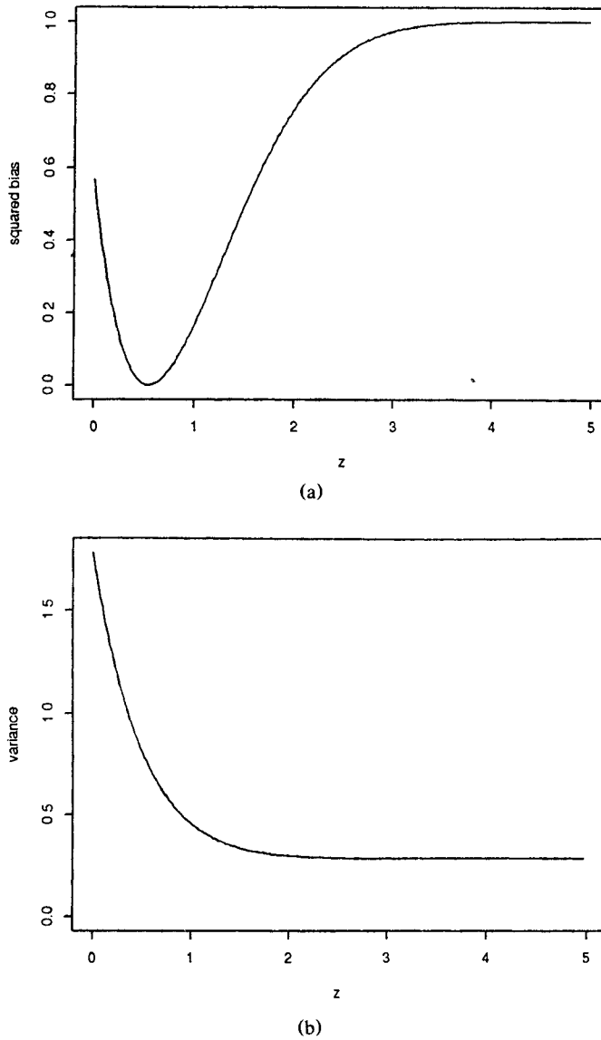
FIG. 1. Normal kernel.
