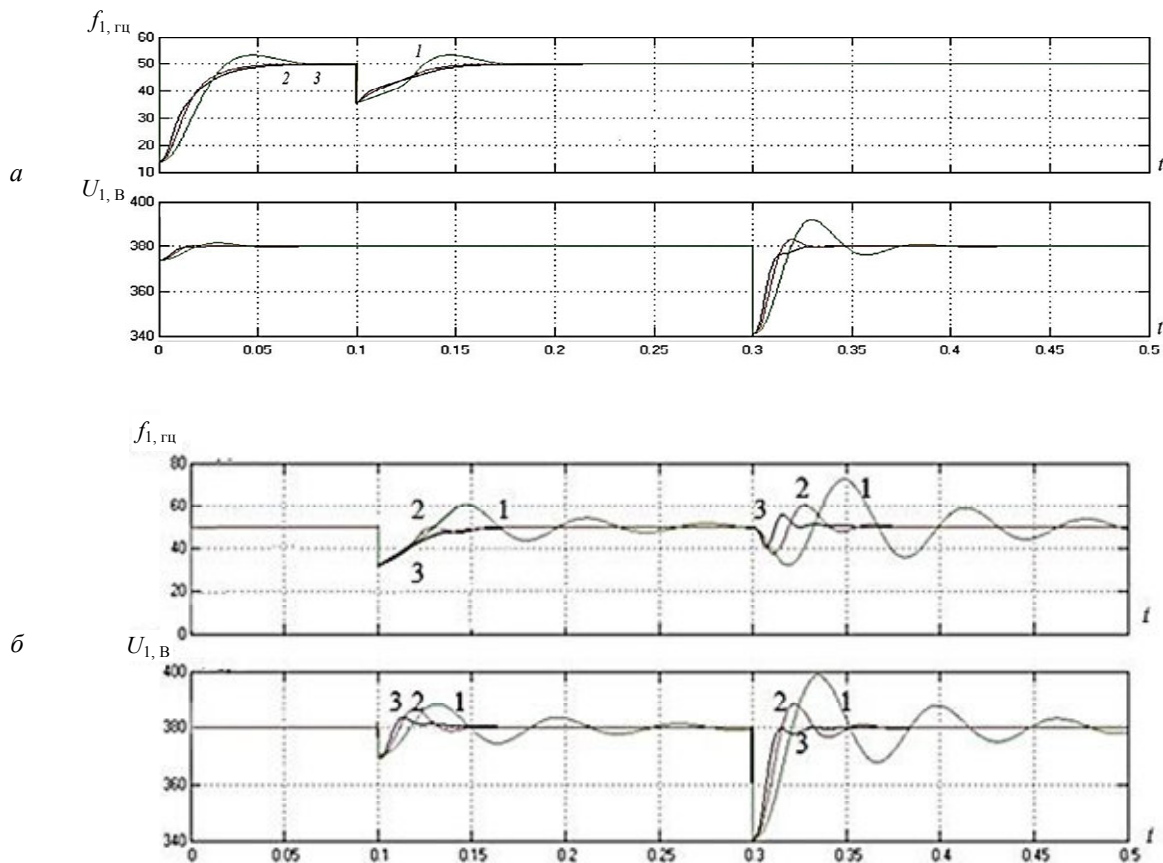
Рис. 4. Зависимости U_1(t) и f_1(t) при подключении нагрузки S_{ном} = P_{ном}(\cos\varphi_{наг} = 1) , t = 0,1 с; S_{ном} = Q_{ном}(\cos\varphi_{наг} = 0) , t = 0,3 с; 1 – s_{настр} = 0,2 ; 2 – s_{настр} = 0,5 ; 3 – s_{настр} = 1 ; а – без учета перекрестных связей; б – с учетом перекрестных связей
