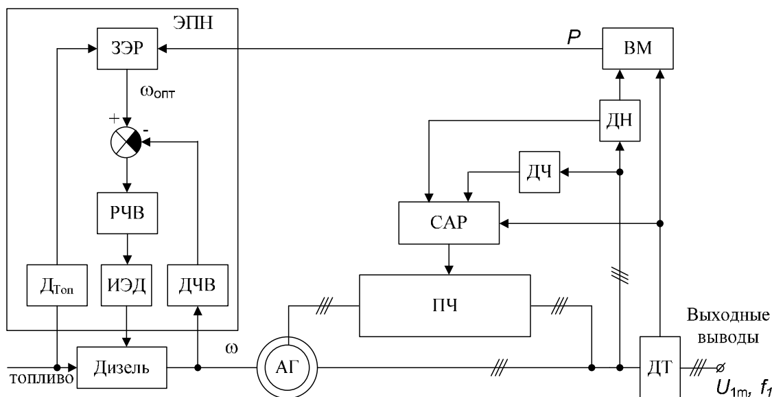
Рис. 1. Функциональная схема вентильной дизель-генераторной электростанции по схеме МДП:
