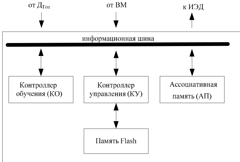
Рис. 2. Функциональная схема ЗЭР
