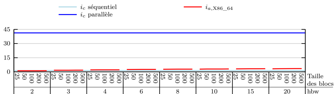
Figure 6.5 : Comparaison entre i_a et les intensités arithmétiques critiques de _{1 \times 4}^{32} SandyBridge.
