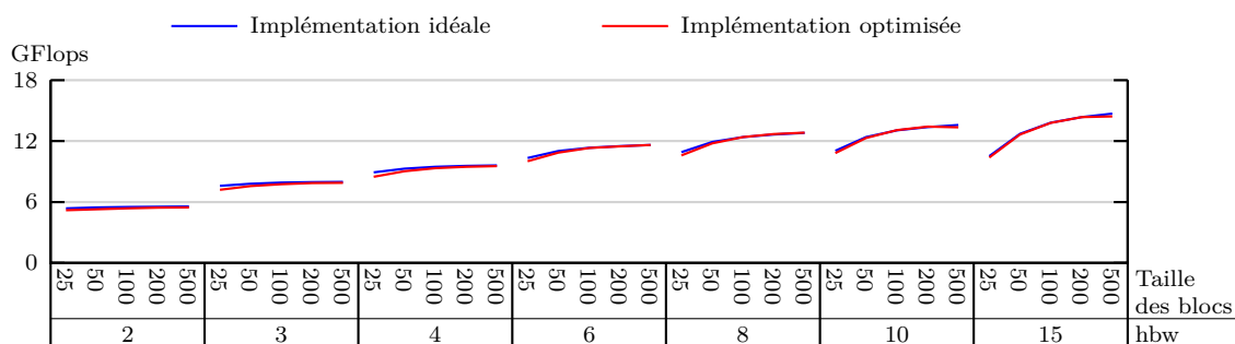
Figure 6.10 : Performances de l'implémentation optimisée sur 1 \times 4 SandyBridge (exécution parallèle).
