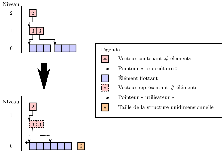
Figure 5.2 : Sériailisation des données d'une structure à deux niveau.
