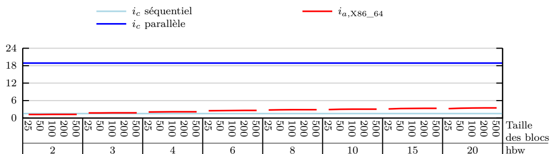
Figure 6.4 : Comparaison entre i_a et les intensités arithmétiques critiques de _{2 \times 4}^{32} Nehalem.
