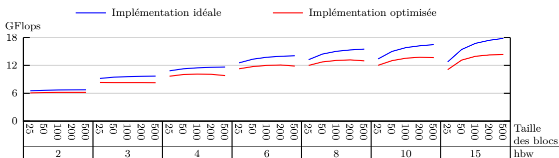
Figure 6.9 : Performances de l'implémentation optimisée sur 2 \times 4 Nehalem (exécution parallèle).
