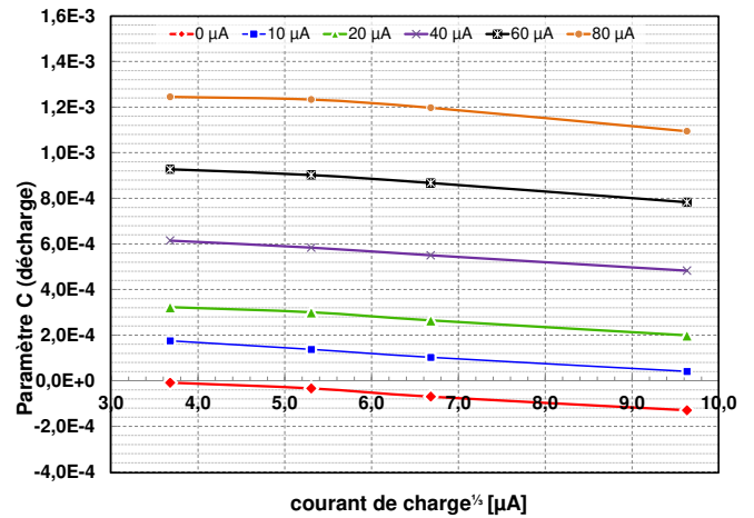
Fig. 96 – régression linéaire du paramètre C en décharge, en fonction de la racine cubique du courant de charge.
