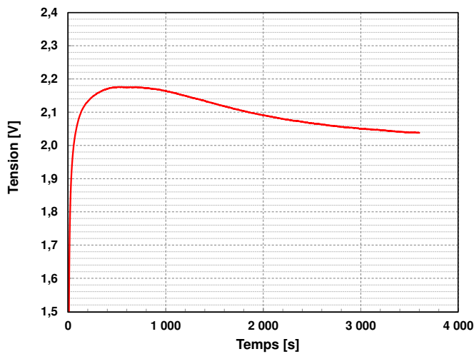
Fig. 84 – évolution du potentiel d'un micro-supercondensateur chargé à 10 \mu\text{A} (constant).
