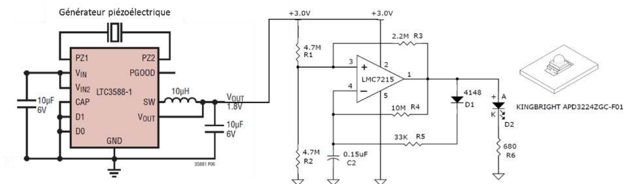
Fig. 82 – schéma électrique du circuit de validation expérimentale visuelle.
