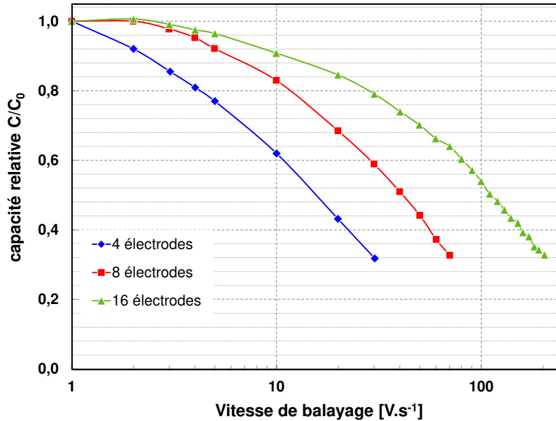
Fig. 75 – capacité normalisée 86 ( C/C_0 ) en fonction de la vitesse de balayage pour des microstructures différentes (4 à 16 électrodes interdigitées). Ici les oignons de carbone constituent le matériau d'électrode (7 \mu m d'épaisseur).
