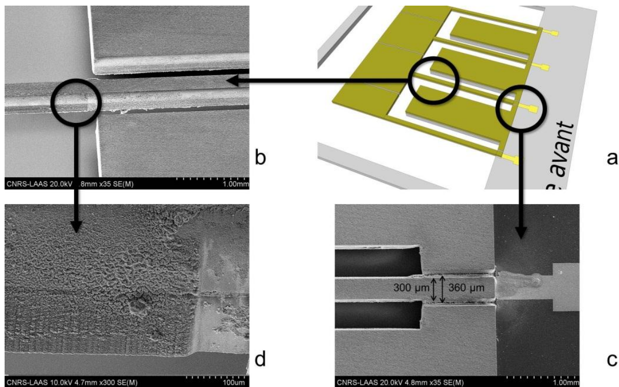
Fig. 32 – b) image MEB d'une des poutres après découpe LASER ; c) grossissement sur le flanc de la poutre : observer le redépôt ; d) vue de dessus de la poutre à l'encastrement pour confirmer les mesures profilomètre LASER confocal ; toutes les vues sont repérées sur le schéma a).
