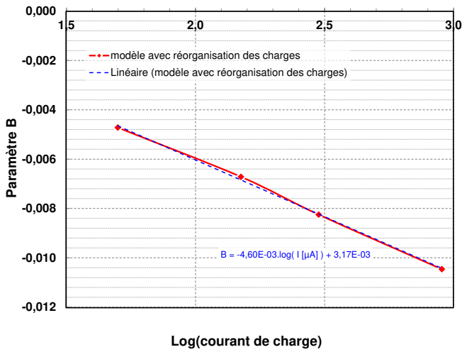
Fig. 93 – régression linéaire du paramètre B en charge, en fonction du logarithme (base 10) du courant.
