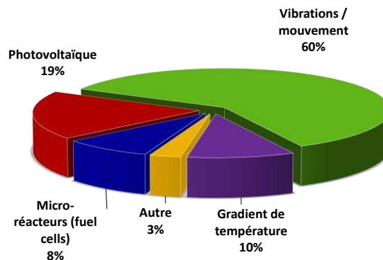
Fig. 11 – Nature des sources d'énergie pour microsystèmes autonomes dans les 10 articles de synthèse publiés entre 2005 et 2009. La récupération d'énergie à partir des vibrations domine, notamment parce que c'est une source très courante aux abords d'une activité « humaine » (au sens large : trafic routier, machines, mouvements).
