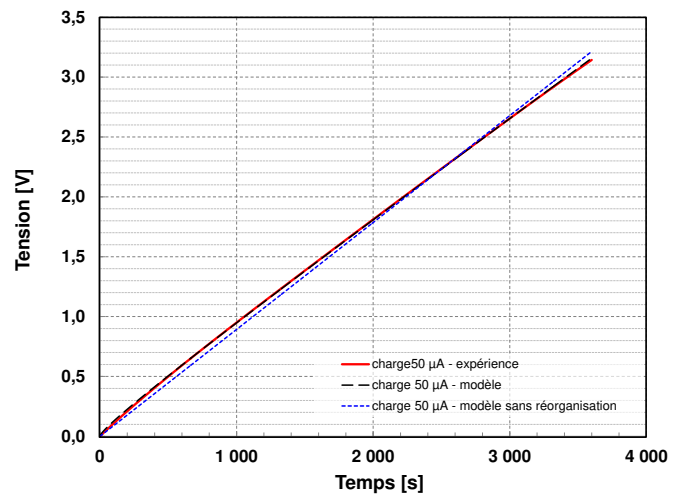
Fig. 92 – évolution du potentiel d'un supercondensateur commercial (50 mF) chargé 50 µA (constant), et la modélisation associée (modèle avec réorganisation de charges et sans réorganisation de charges).
