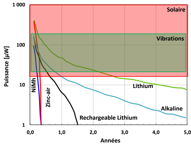
Fig. 10 - Comparaison de la puissance disponible au cours des années selon la source d'énergie, d'après [38].
