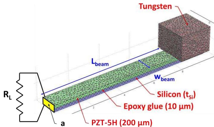
Fig. 23 - modèle éléments finis/SPICE
