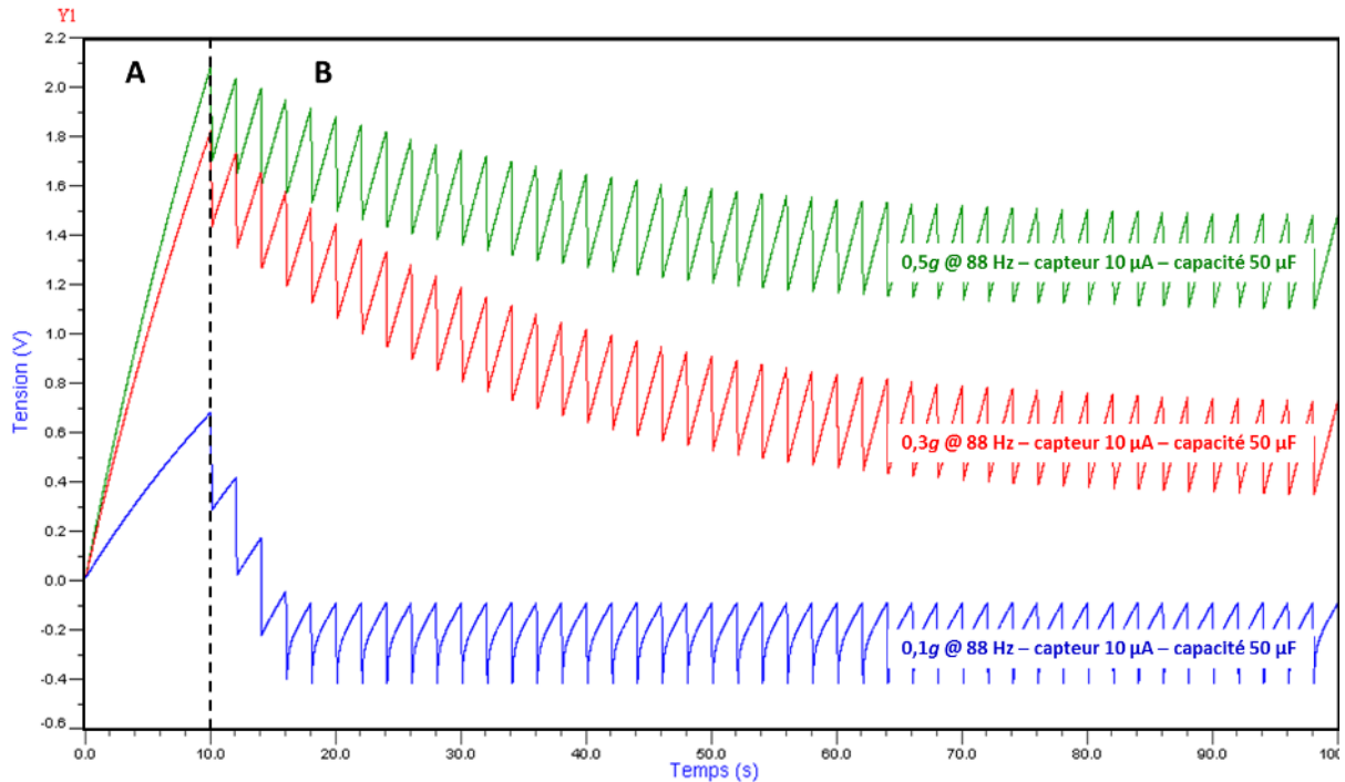
Fig. 98 – évolution du potentiel du dispositif de stockage (condensateur 10 \mu\text{F} ). Il n'y a pas de consommation du capteur pendant les 10 premières secondes (zone A) ; celle-ci est fixée à 10 \mu\text{A} en moyenne ensuite (pulsations de 100 \mu\text{A} pendant 100 ms toutes les 1 s). Le micro-générateur piézoélectrique alimente le système à partir de vibrations de 0,1g, 0,3g et 0,5g.
