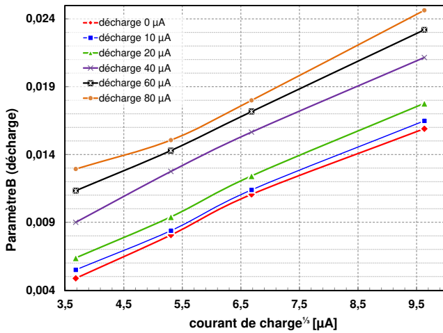
Fig. 95 – régression linéaire du paramètre B en décharge, en fonction de la racine cubique 94 du courant de charge.
