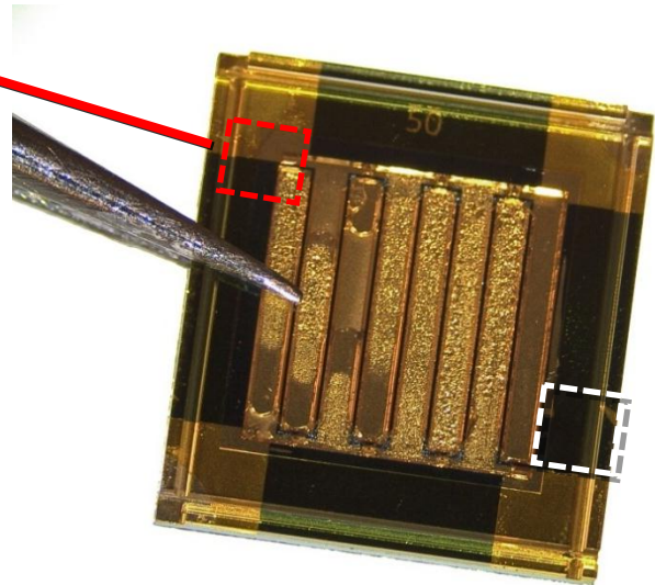
Fig. 67 – électrolyte (carbonate de propylène) encapsulé dans des cuves de 104\ \mu\text{m} de profondeur. La zone repérée par un carré pointillé blanc correspond à la zone étudiée dans Fig. 69.
