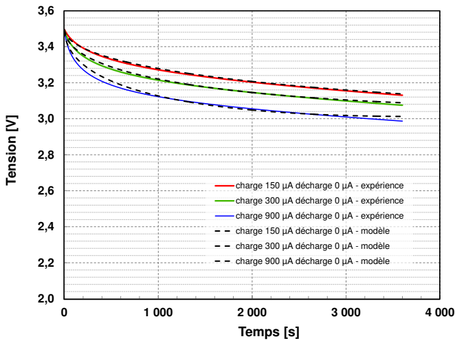
Fig. 89 – évolution du potentiel d'un supercondensateur commercial (50 mF) chargé à différents courant (constants), puis laissé en circuit ouvert), et la modélisation associée (modèle avec réorganisation de charges).
