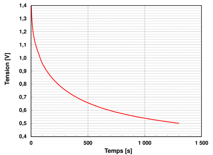
Fig. 85 – évolution du potentiel d'un micro-supercondensateur en circuit ouvert après une charge à 10 \mu\text{A} (constants) jusqu'à 2,05 V.
