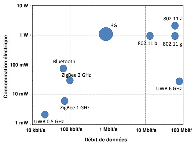
Fig. 8 - consommation des différents protocoles de communication radio par rapport au débit de données. D'après [26].
