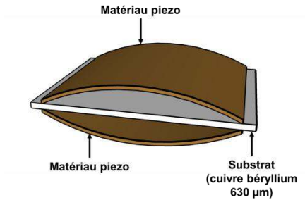
Fig. 20–dispositif de récupération d'énergie à partir de vibrations au format cymbale, d'après [33].
