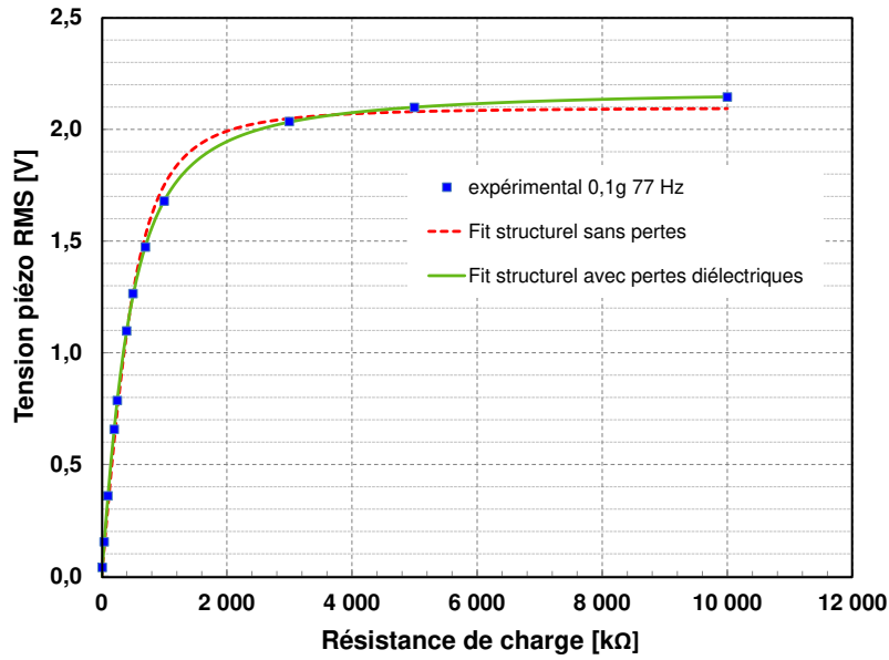
Fig. 88 – caractéristique tension/résistance du modèle structurel avec et sans pertes diélectriques (modélisées par la résistance parallèle R_p sur la Fig. 86) par rapport aux données expérimentales (0,1g à 77 Hz).
