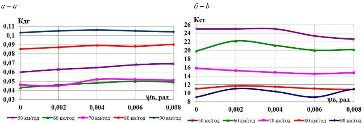
Рис. 6. Графіки зміни динамічних показників від швидкості руху: a – максимального відношення рамної сили до статичного осьового навантаження; б – коефіцієнта стійкості від сходження колеса з рейок
