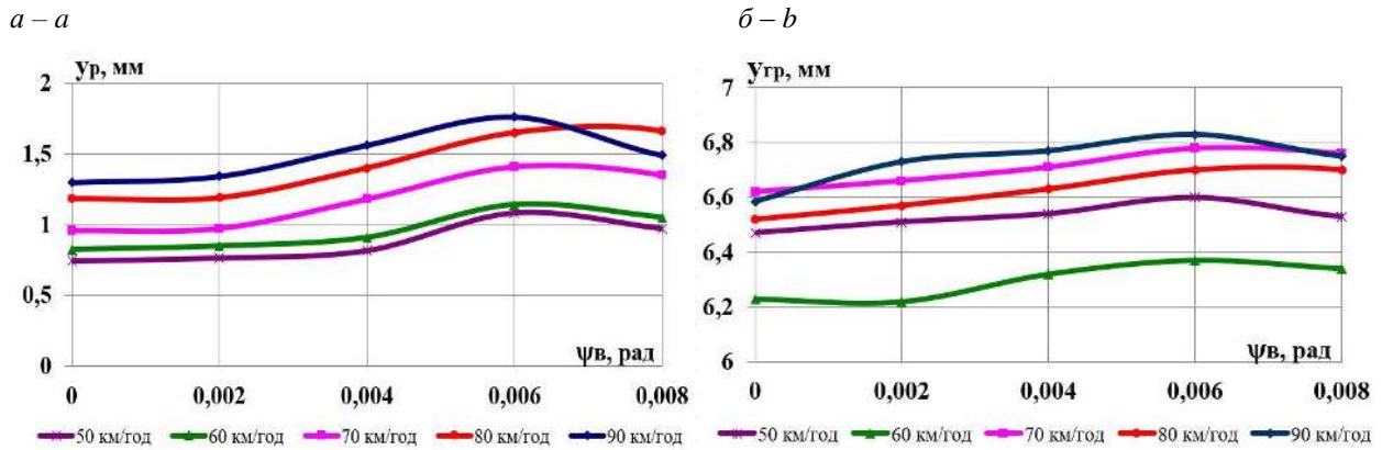
Рис. 10. Графіки зміни динамічних показників від швидкості руху: а – відтискання підшви рейки; б – відтискання головки рейки
