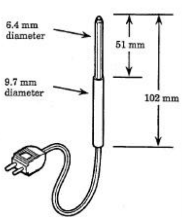
Fig. 1. Hg pencil-type discharge lamp.
