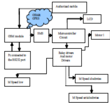
Fig 1.6:Wireless communication of IM
