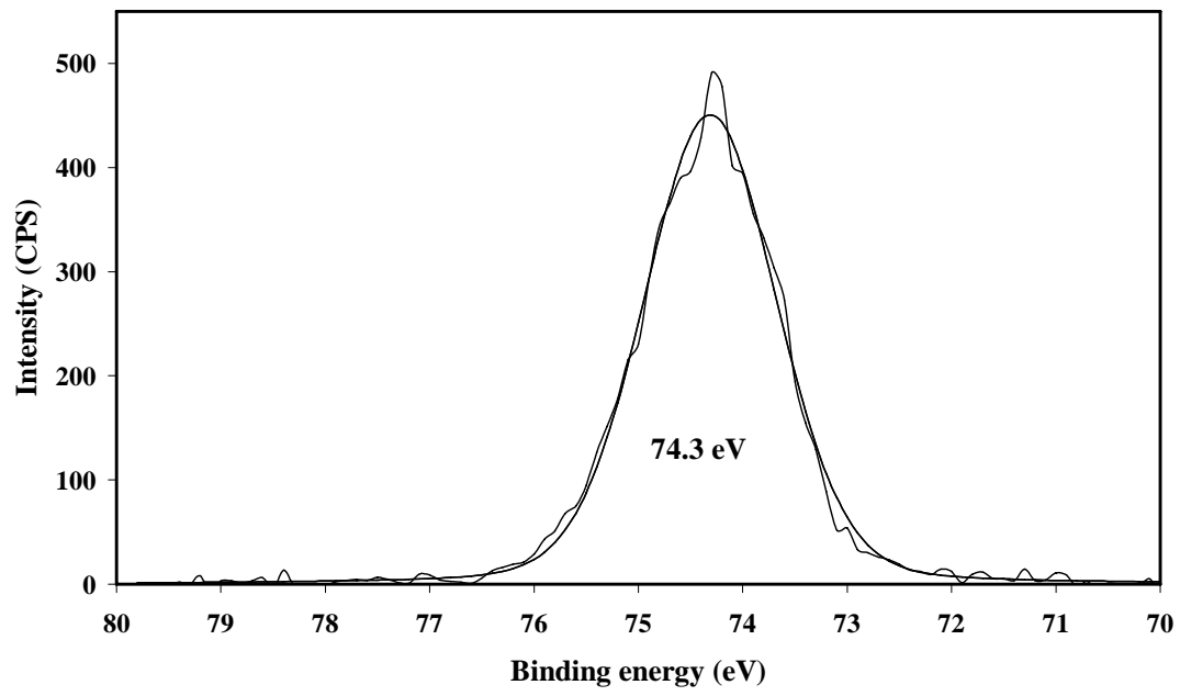
Fig. 2e Al 2p pseudoboehmite
