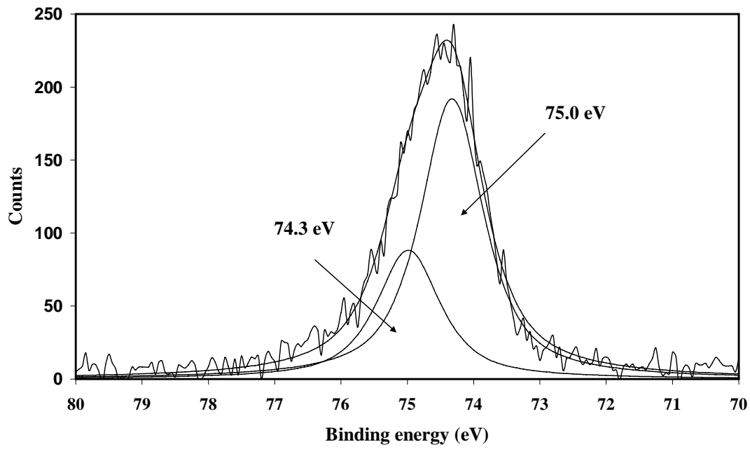
Fig. 2c Al 2p bayerite
