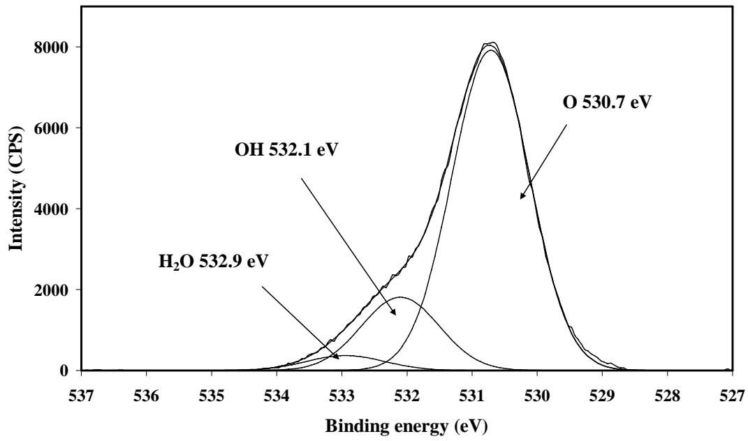
Fig. 1a O 1s corundum
