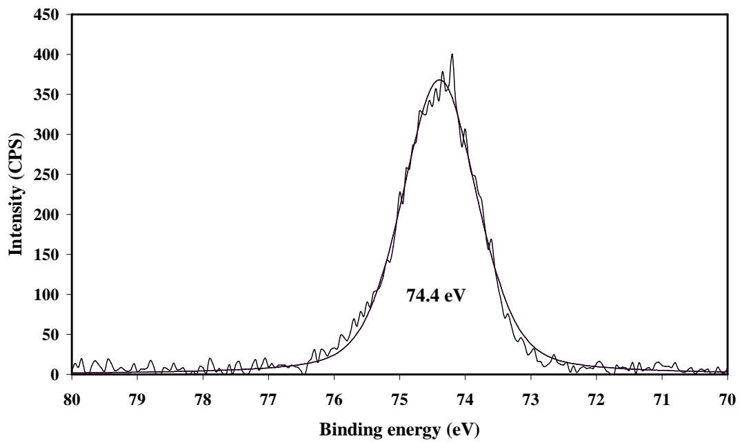
Fig 2b Al 2p gibbsite
