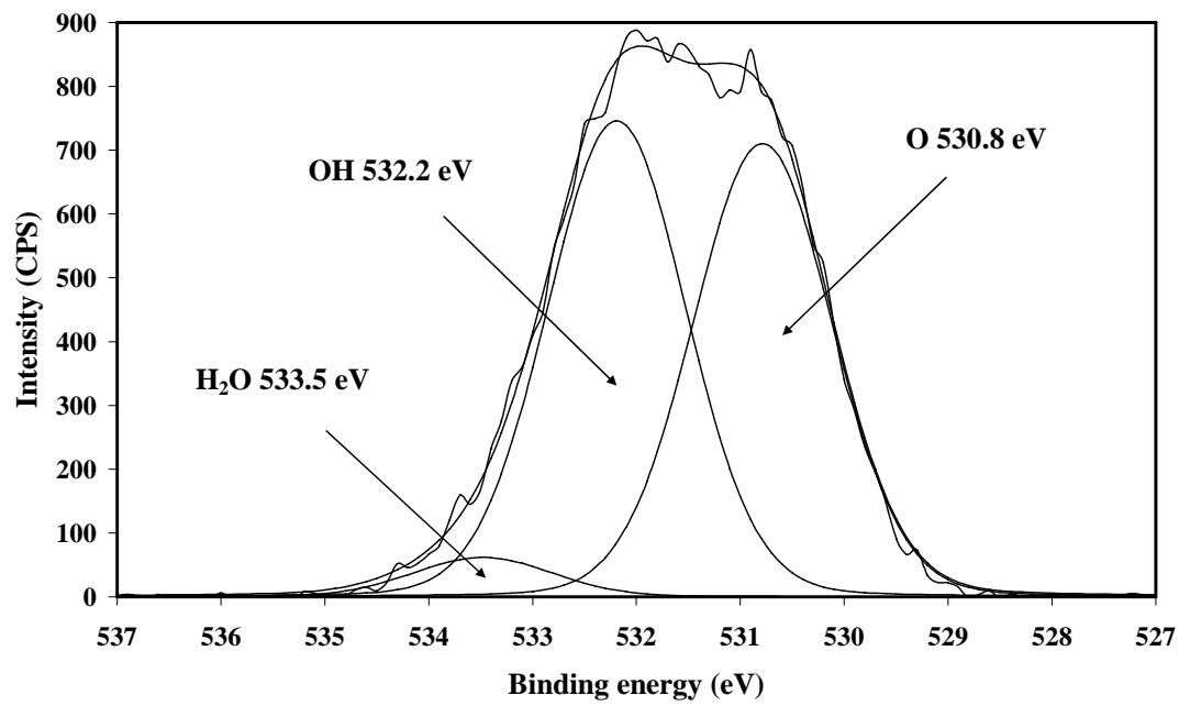
Fig. 1e O 1s pseudoboehmite
