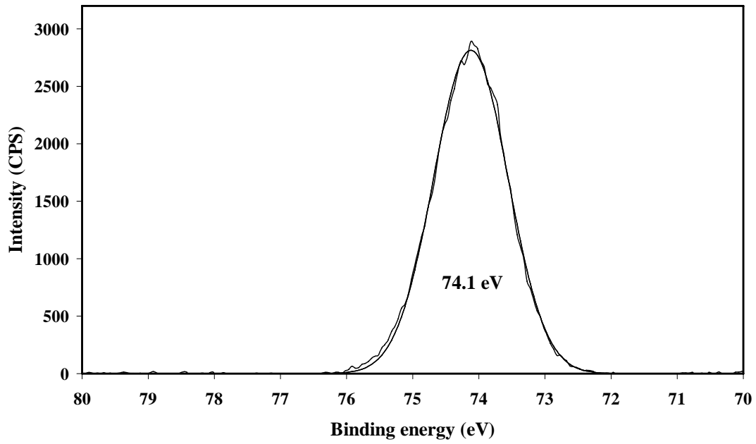
Fig. 2a Al 2p corundum
