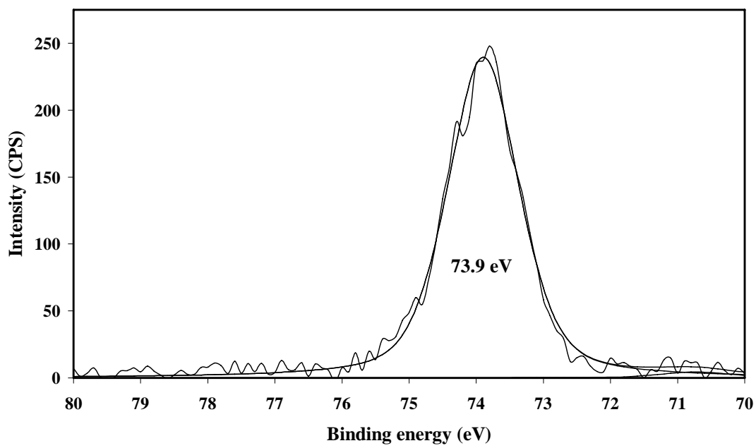
Fig. 2d Al 2p boehmite
