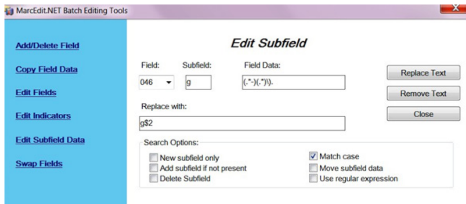
Rys. 1. Przykład, w jaki sposób można użyć narzędzia 'Edit Subfield' ('Edytuj Podpole') w MarcEdit do edycji danych w procesie ekstrakcji
