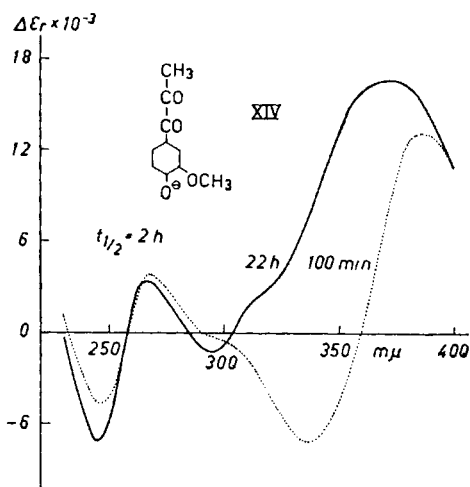
Fig. 7. \Delta\epsilon_r -Kurven für Vanillylmethylketon (XIV) nach verschiedenen Reduktionszeiten.
