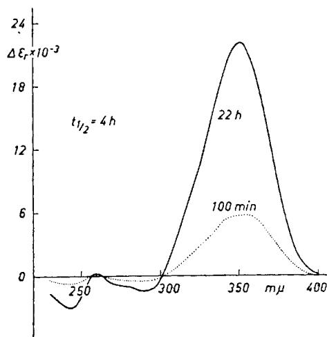
Fig. 5. \Delta\epsilon_r -Kurven für \alpha -Oxy-propioquajakon (XI) nach verschiedenen Reduktionszeiten.
