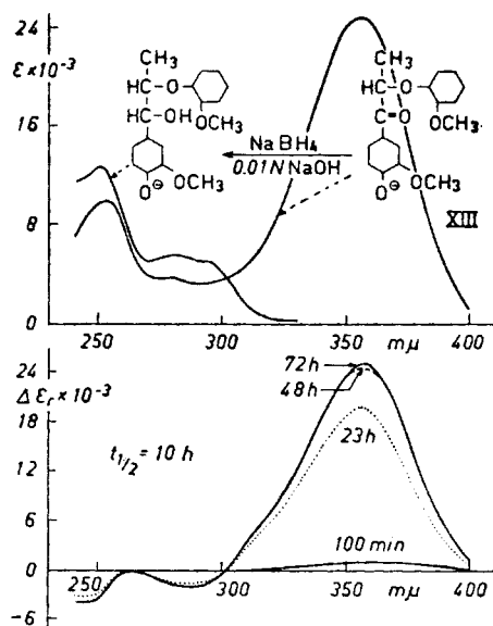
Fig. 6. Oben: Absorptionskurven von \alpha -Guajakoxy-propionguajakon (XIII) und dessen Borhydridreduktionsprodukt (72 h Reduktionsdauer). Unten: \Delta\epsilon_r -Kurven nach verschiedenen Reduktionszeiten.
