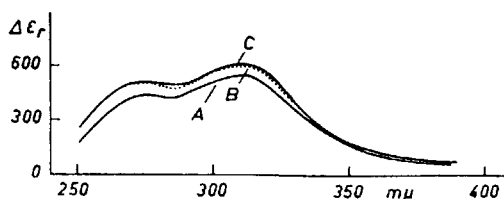
Fig. 15. \Delta\epsilon_r -Kurven eines mit \text{CH}_3\text{N}_3 methylierten Björkman-Lignins (DL III) nach 100 min (A), 22 h (B) und 46 h (C) Reduktionsdauer.
