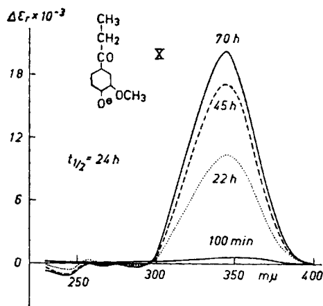
Fig. 4. \Delta\epsilon_r -Kurven für 4-Propioguajakon (X) nach verschiedenen Reduktionszeiten.
