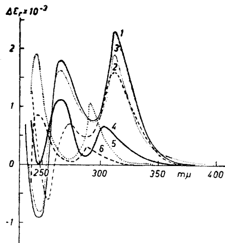
Fig. 10. \Delta\epsilon_r -Kurven für 1) Guajacylaceton (XXII); 2) Syringylaceton (XXIV); 3) \omega -Oxyguajacylaceton (XXV); 4) 4-Oxy-2,6-dimethoxyphenylaceton (XXVI); 5) Veratrylaceton (XXIII); 6) 2,4,6-Trimethoxyphenylaceton (XXVII), nach 100 min Reduktionsdauer.
